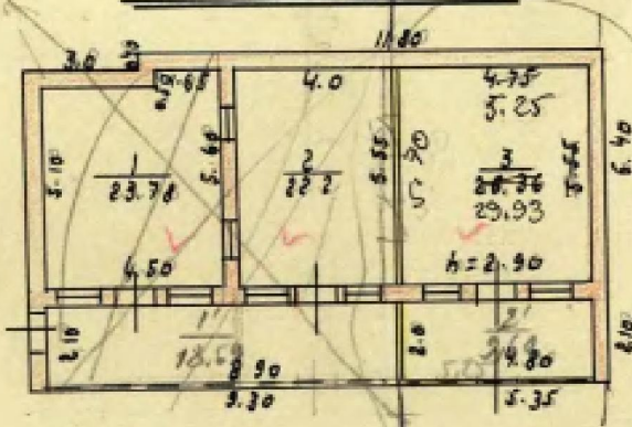
План 2 го I этаж
