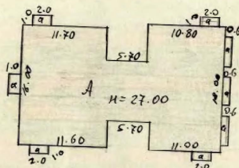
ГЕН-ПЛАН
